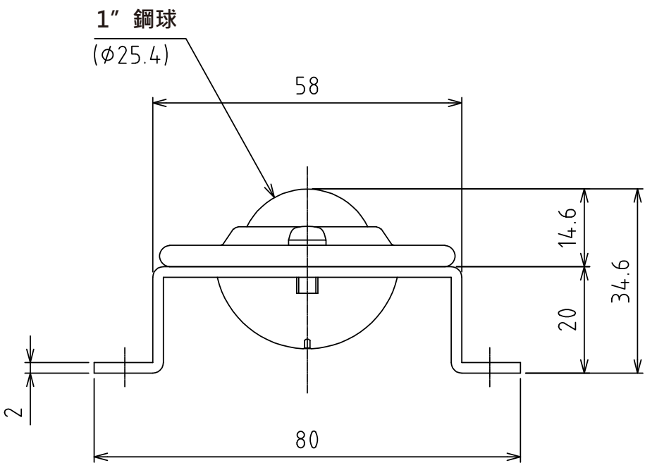
A視圖 (尺度 1:1)
