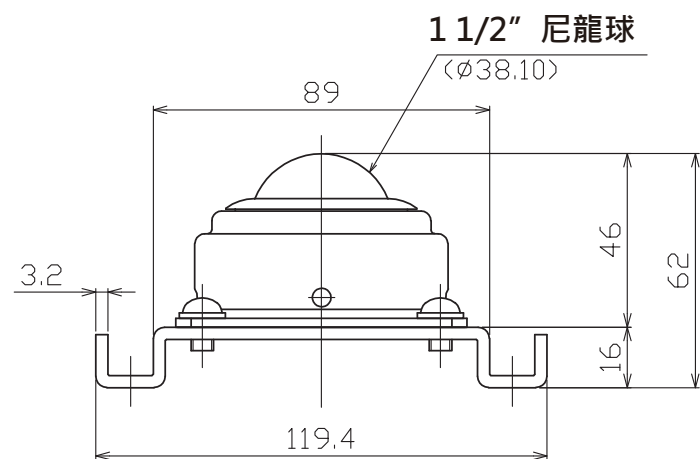
A視圖 (尺度 1:3)
