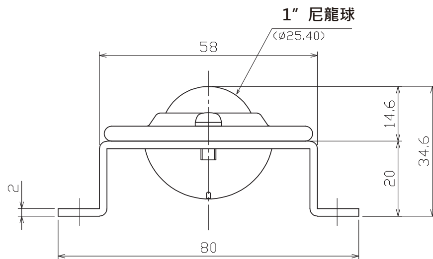
A視圖 (尺度 1:1)
