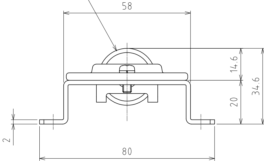
A視圖
