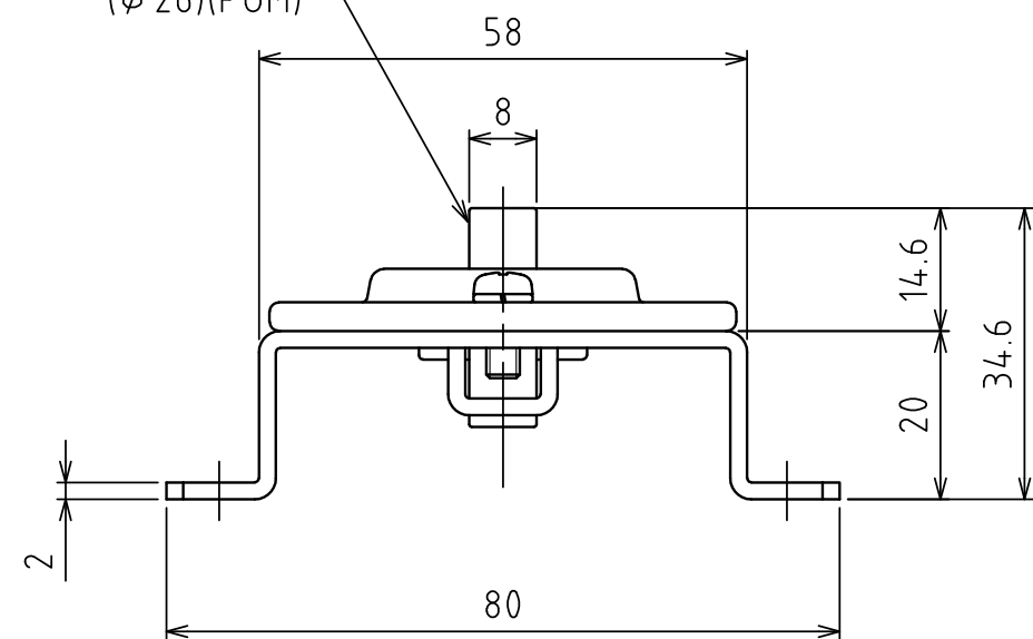
A視圖 (尺度 1:1)
